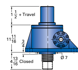
75-MSJ-I INVERTED
