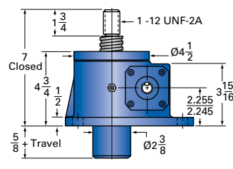
5-MSJ-U UPRIGHT
