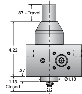
0.5C-BSJ-I & 0.5CHL-BSJ-I INVERTED
