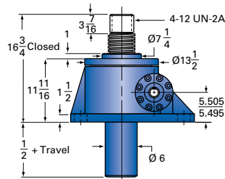
75-MSJ-U UPRIGHT
