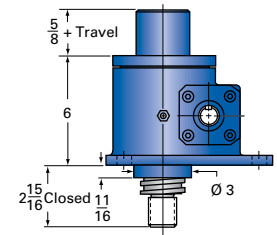
15-MSJ-I INVERTED
