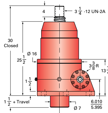
100-BSJ-U UPRIGHT
